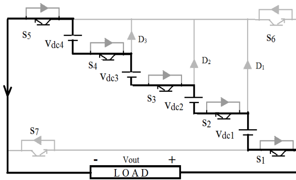
(d) V_{out} = -V_{dc4} - V_{dc3} - V_{dc2} - V_{dc1}
